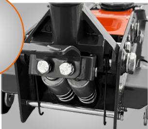
› Quick-Lift Funktion durch Doppelkolben
