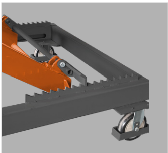
› Sicherheitsrastung schützt vor ungewolltem Ablassen
