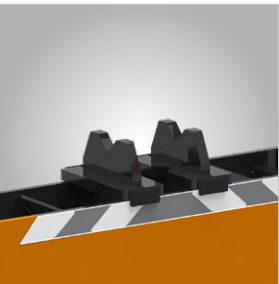
Patentiertes Führungssystem garantiert optimale Positionierung der Prismenblöcke
